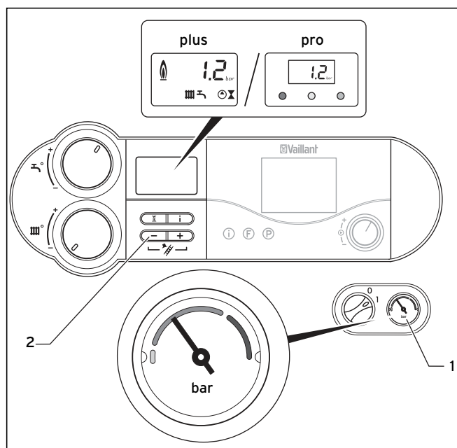
6.1 ábra Fűtési rendszer töltési nyomása ellenőrzése
