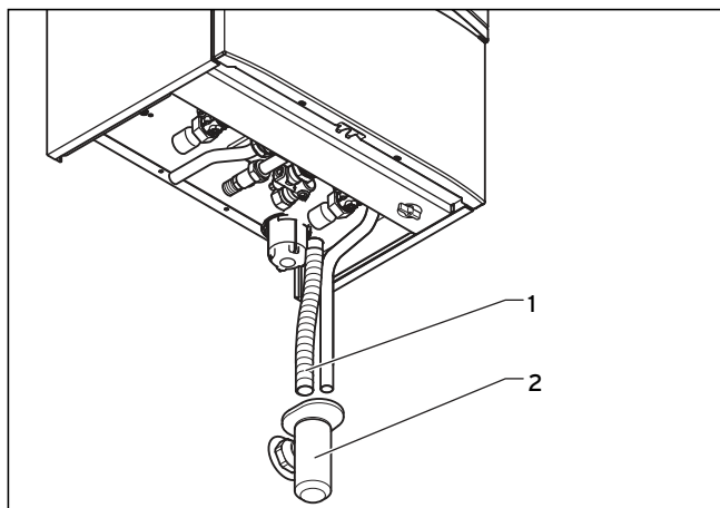
5.8 ábra Kondenzvízkifolyó
