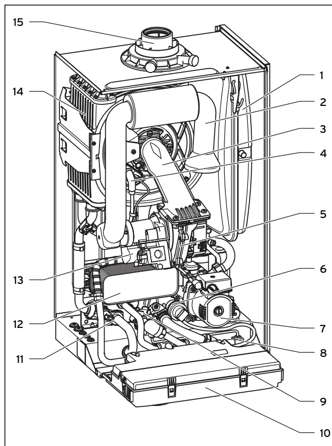
2.1 ábra VUW INT funkcionális elemei
