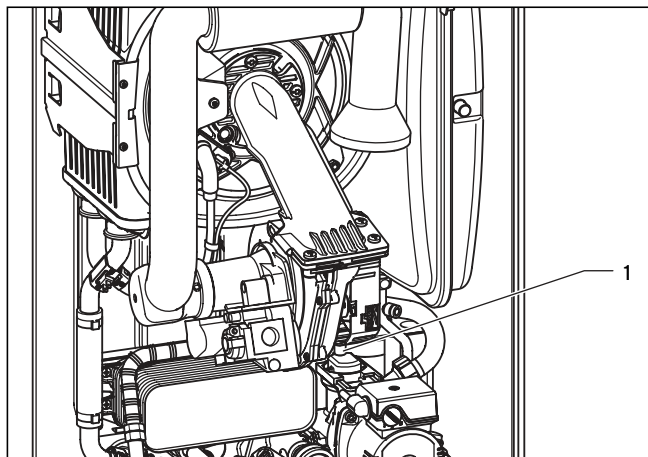
6.2 ábra Gyorslégtelenítő
