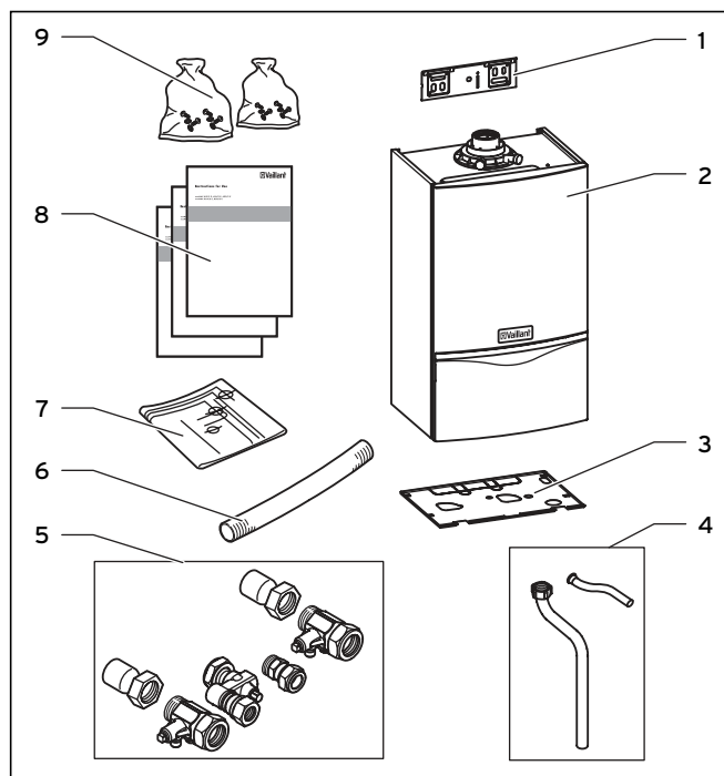
4.1 ábra A VUW-készülékek szállítási terjedelem (csak ecoTEC plus készülékek)
