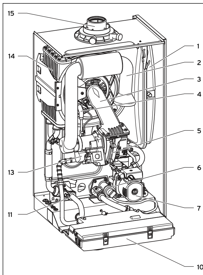
2.2 ábra VU INT funkcionális elemei
