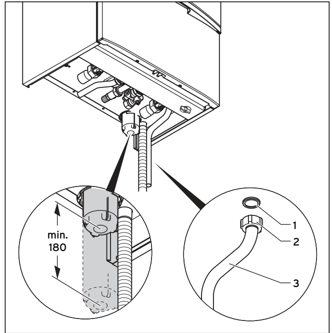
5.6 ábra Lefolyócső szerelése a biztonsági szelepre (példa: VUW-készülék)
