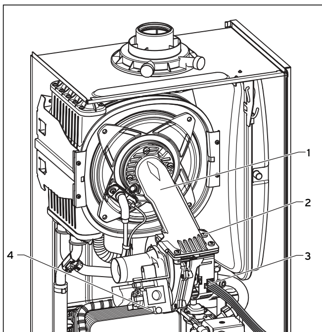
10.2 ábra Gázarmatúras ventilátor kicserélése
