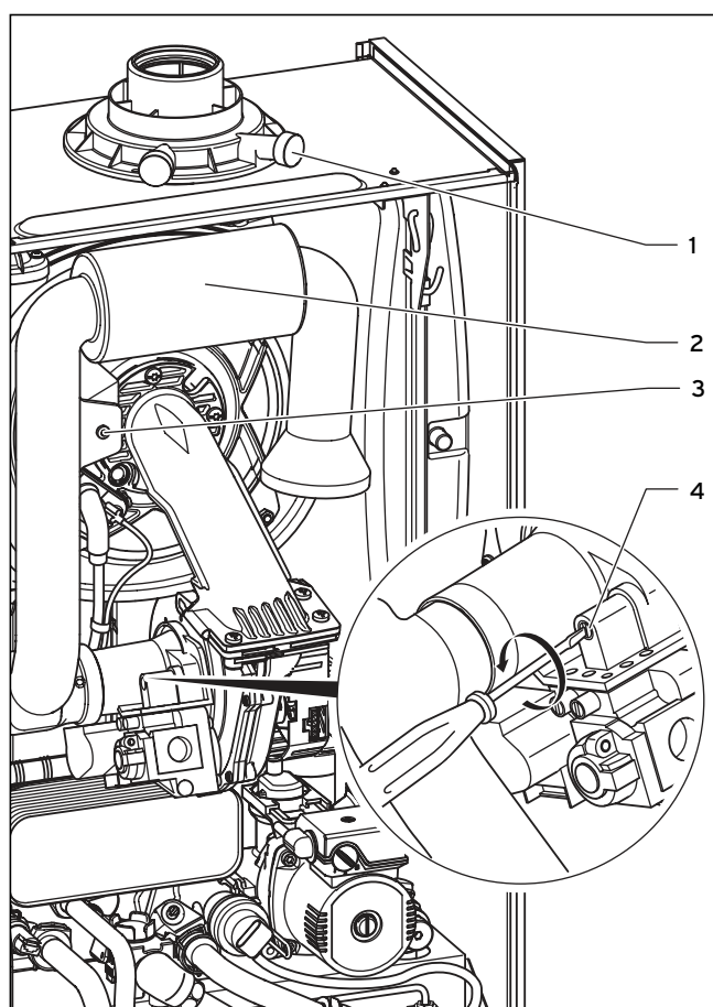
6.5 ábra CO 2 -mérés és a légellátási tényező beállítása (gázbeállítás)
