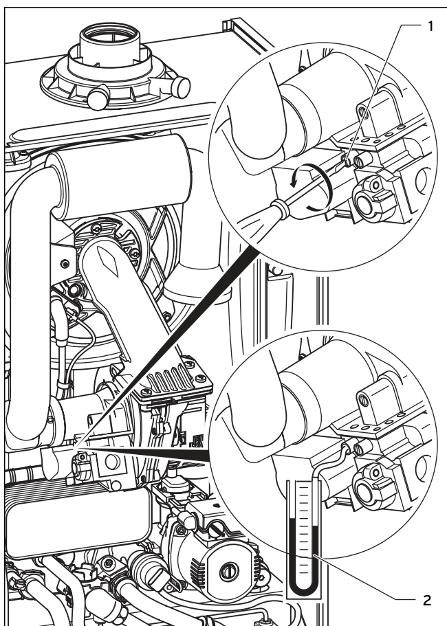
6.4 ábra Mérje meg a csatlakozási gáznyomást
