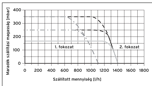
7.2 ábra Szivattyú-jelleggörbe
