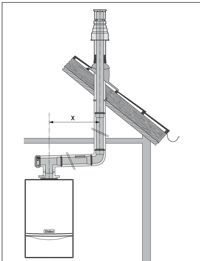
5.7 ábra Szerelési példa: Függőleges tetőátvezető
