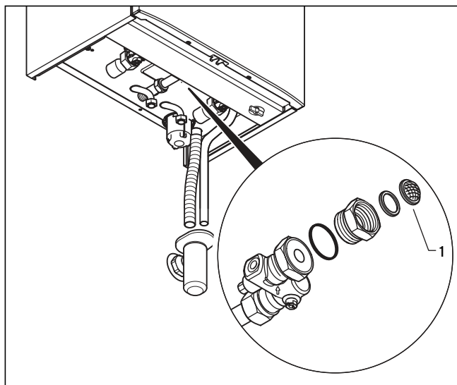
8.9 ábra A hidegvíz-bevezetésben lévő szűrő kiserelése
