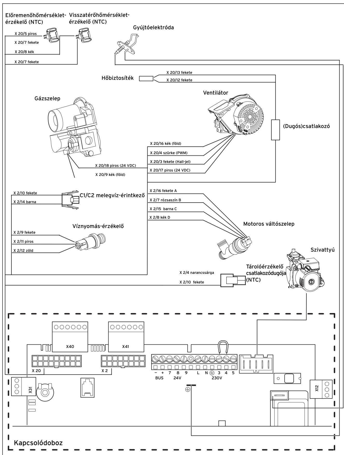
5.13 ábra Kábelösszefűgési terv, ecoTEC VU készülék
