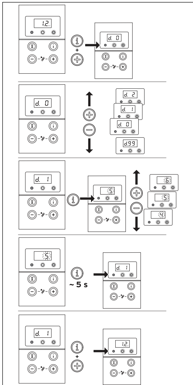
7.1 ábra Paraméterek beállítása
