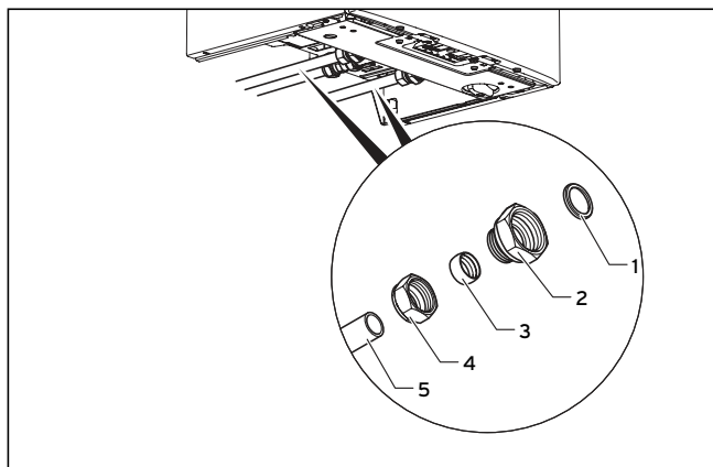
5.2 ábra Hideg- és melegvízcsatlakozó felszerelése (példa)
