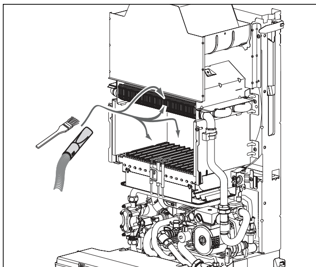
8.1 ábra Égő és primer hőcserélő tisztítása az alkatrészek kiserelése nélkül (csekély szennyeződés)
