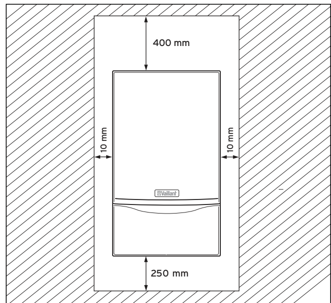
4.3 ábra Szükséges minimális távolságok / szabad szerelési terek
