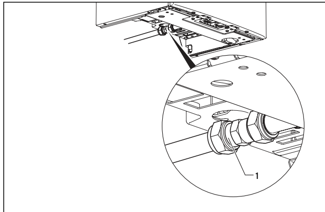
5.1 ábra Gázcsatlakozás
