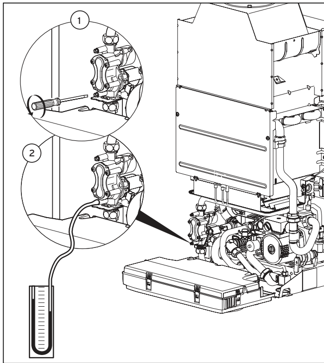
6.3 ábra A csatlakozási nyomás vizsgálata
