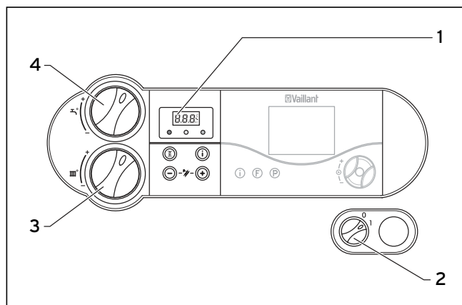
6.2 ábra Fűtési rendszer töltési nyomásának ellenőrzése
