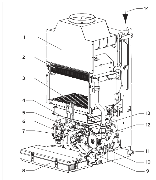
2.1 ábra Funkcionális elemek
