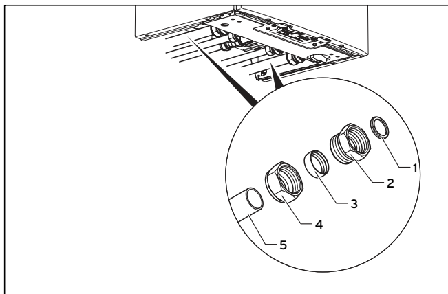
5.3 ábra Fűtési előremenő és fűtési visszatérő csatlakozó felszerelése (példa)
