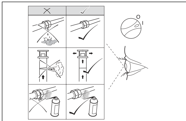
8.4 ábra A működés vizsgálata
