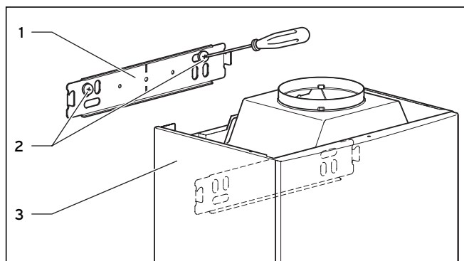
4.5 ábra A készülék felakasztása a falra
