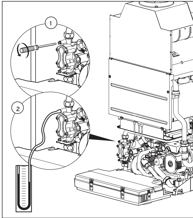
6.4 ábra Névleges terhelés ellenőrzése
