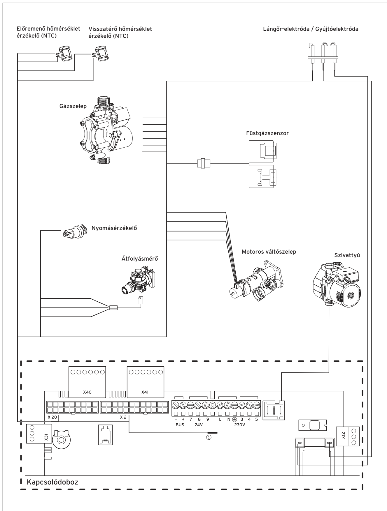
5.8 ábra Az atmoTEC pro kábelösszefüggési rajza
