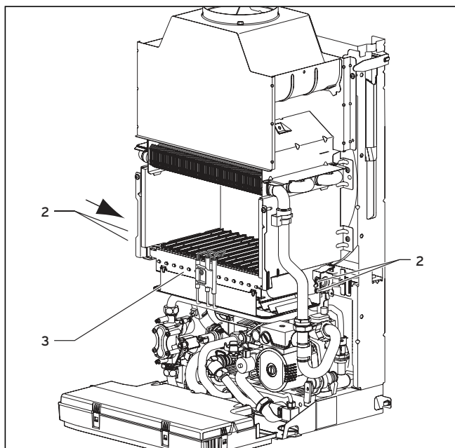
8.3 ábra Égő tisztítása kisereléssel (erősebb szennyeződés)
