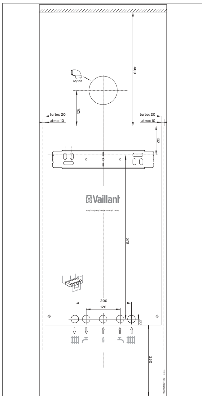
4.4 ábra Szerelőszablon
