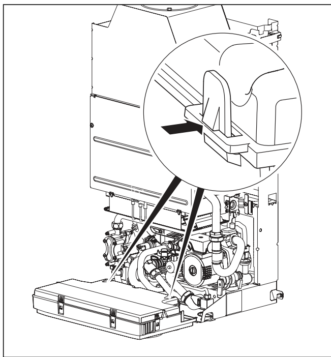
5.5 ábra A kapcsolódoboz hátoldalának kinyitása
