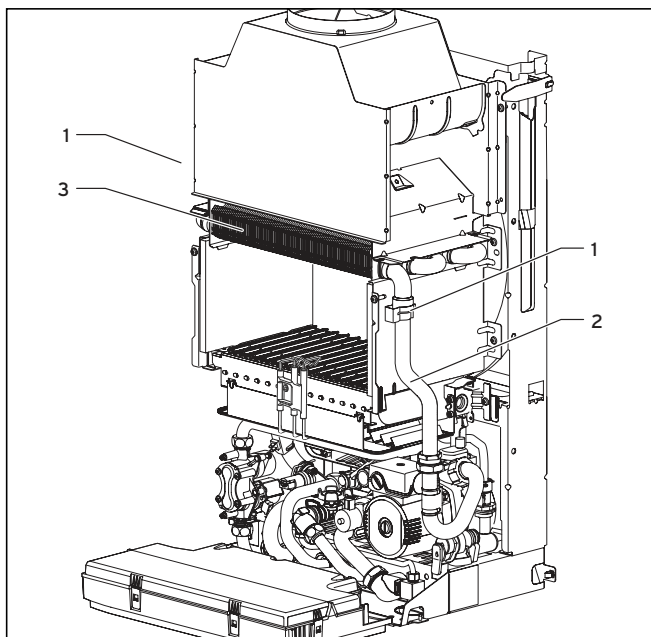
8.2 ábra Primer hőcserélő tisztítása kisereléssel (erősebb szennyeződés)
