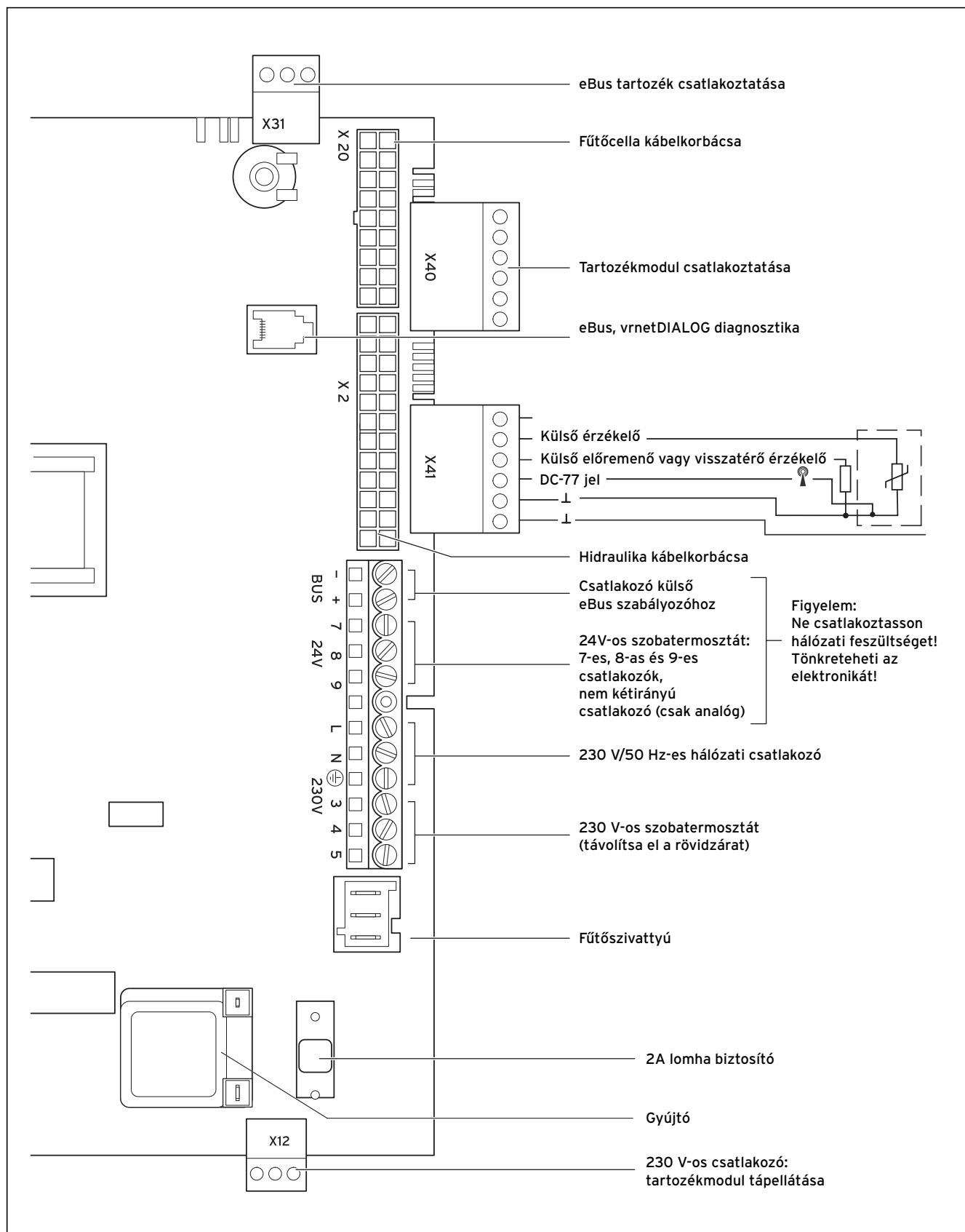
5.7 ábra Az atmoTEC pro bekötési rajza
