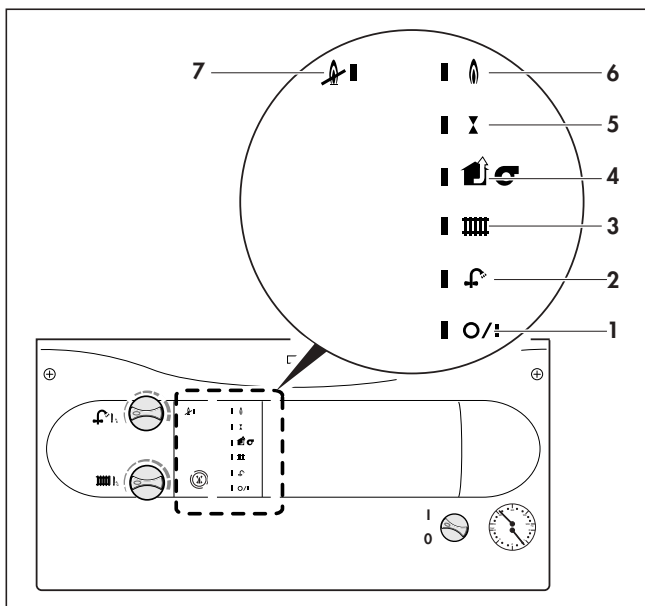
5.2 ábra: Melegvíz és fűtés funkcionális ellenőrzése
