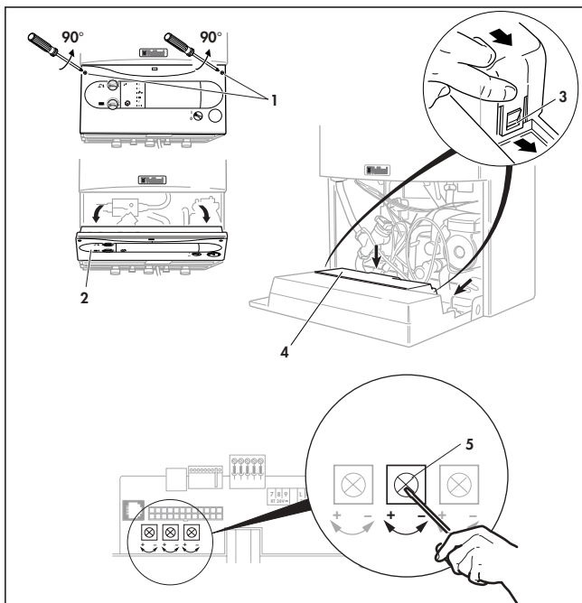
6.2. ábra: Újbóli bekapcsolás tiltásának beállítása fűtési üzemmódhoz
