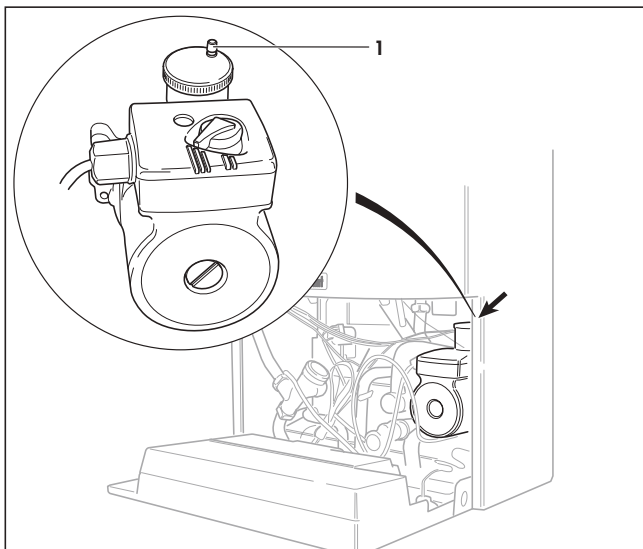
3.16. ábra: Gyorslégtelenítő
