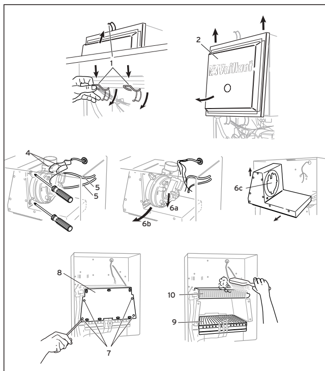
7.1. ábra: A gázégő és a primer hőcserélő tisztítása
