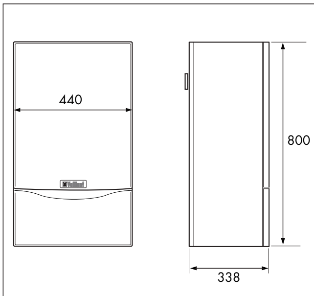
3.4. ábra: A falı gázkészülék fı méretei
