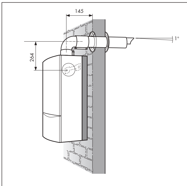
3.12. ábra: Levegő-/fűtőgázvezetés: példa
