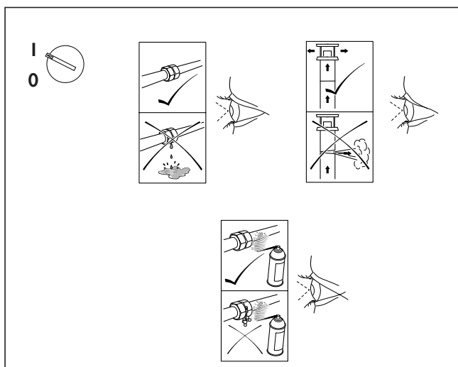
5.1 ábra: Szemrevételezéssel történő vizsgálat
