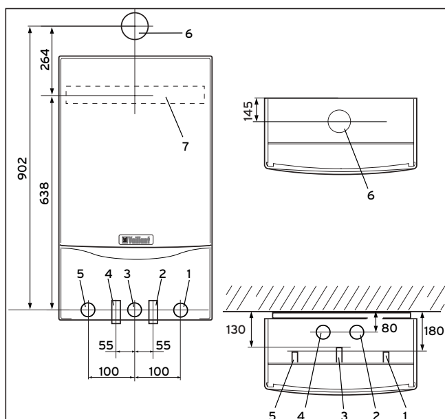
3.6. ábra: Csatlakozási méretek VU
