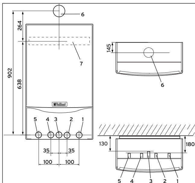
3.5. ábra: Csatlakozási méretek VUW
