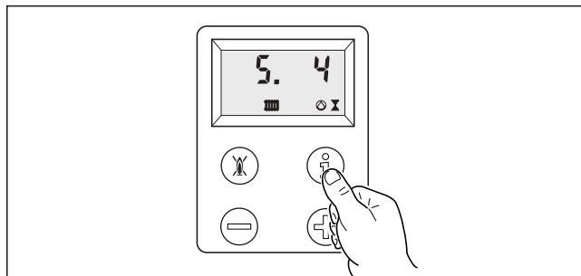
5.3 ábra: Kijelzés fűtés üzemmódban
