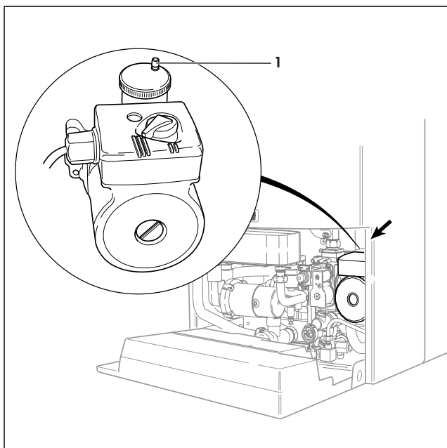
Obr. 3.18: Rychloodvzdušnění Obr. 3.18: Rýchloodvzdušňovač 3.18. ábra: Gyorslégtelenítő
