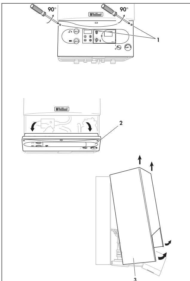
Obr. 3.19: Sejmutí krytu kotle Obr. 3.19: Zloženie krytu prístroja 3.19. ábra: A készülékburkolat levétele
