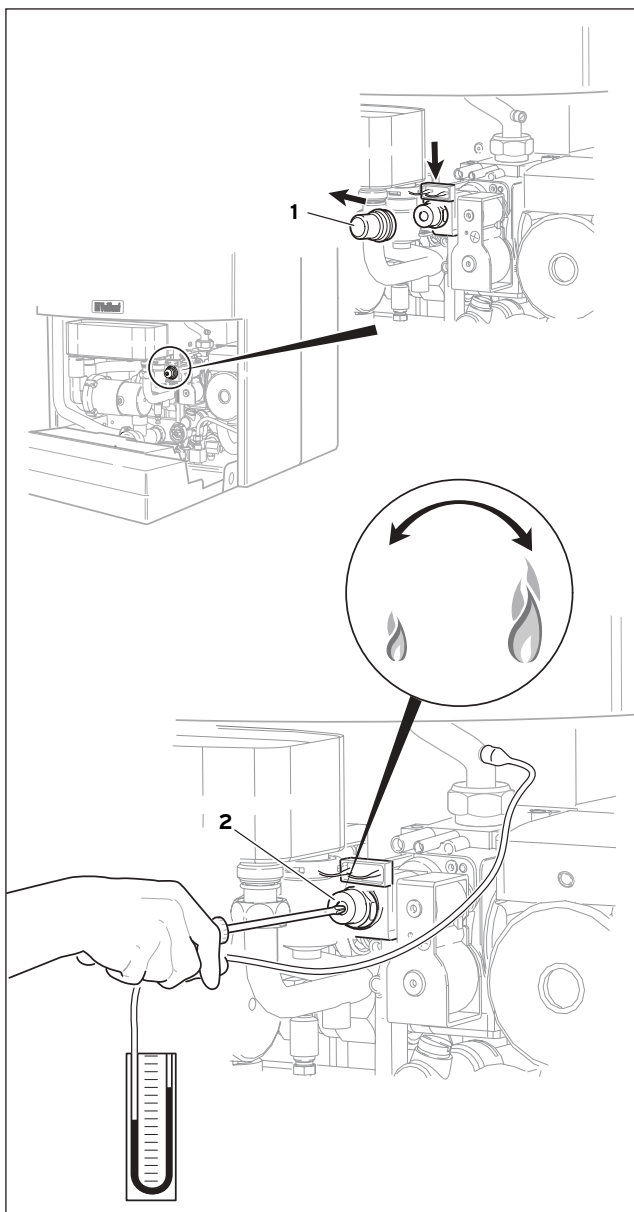
Obr. 4.4: Nastavení startovacího množství plynu Obr. 4.4: Nastavenie zapal'ovacieho množstva plynu 4.4. ábra: A gyújtógáz mennyiségének beállítása
