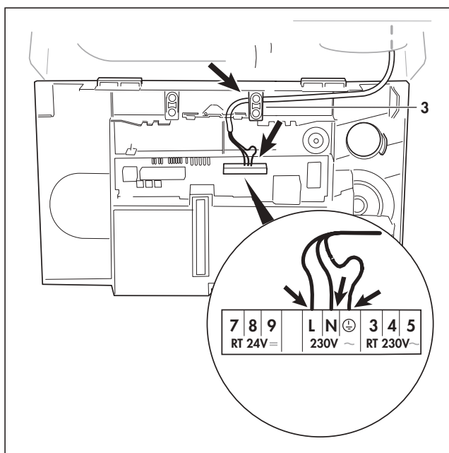
Obr. 3.15: Průchodky pro vedení kabelů Obr. 3.15: Káblový kanál 3.15. ábra: A kábeleket vezetése
