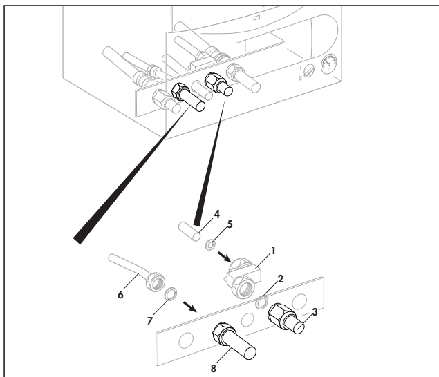
Obr. 3.10: Montáž prípojev studenej a teplej vody SK
