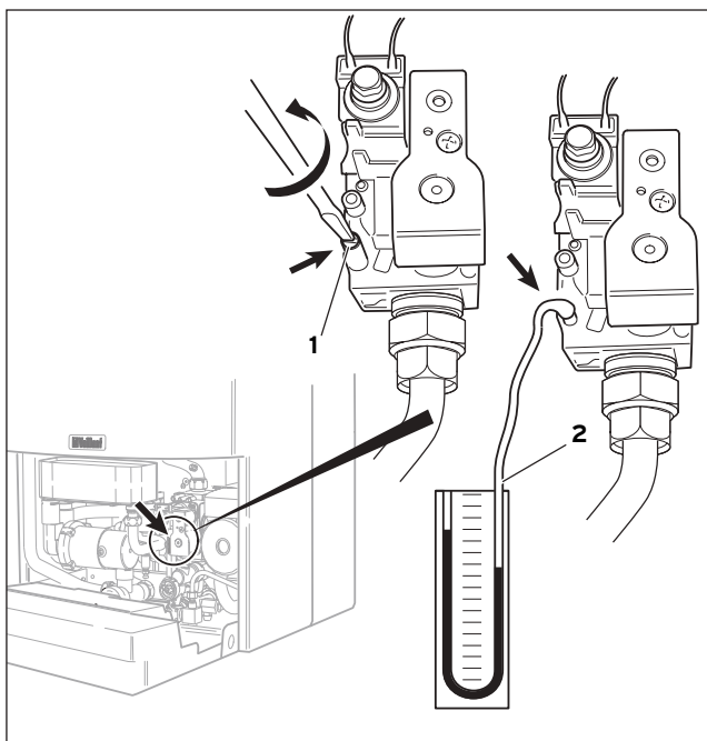
Obr. 5.1: Přezkoušení připojovacího tlaku (průtočného tlaku)
