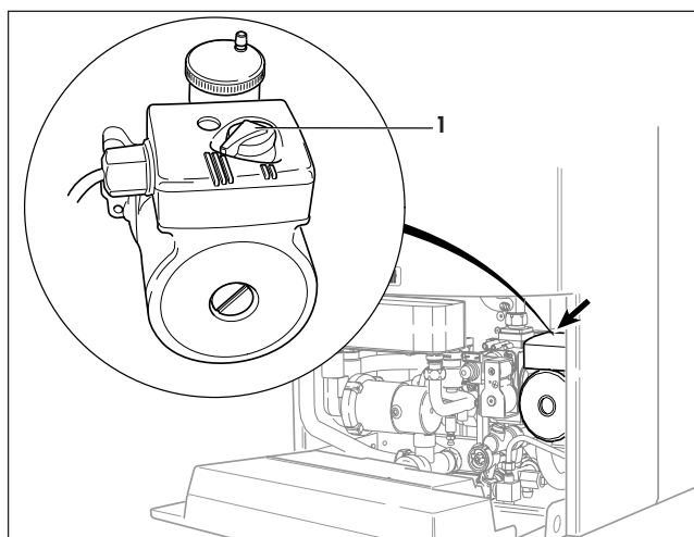
Obr. 7.1: Spínač čerpadla
