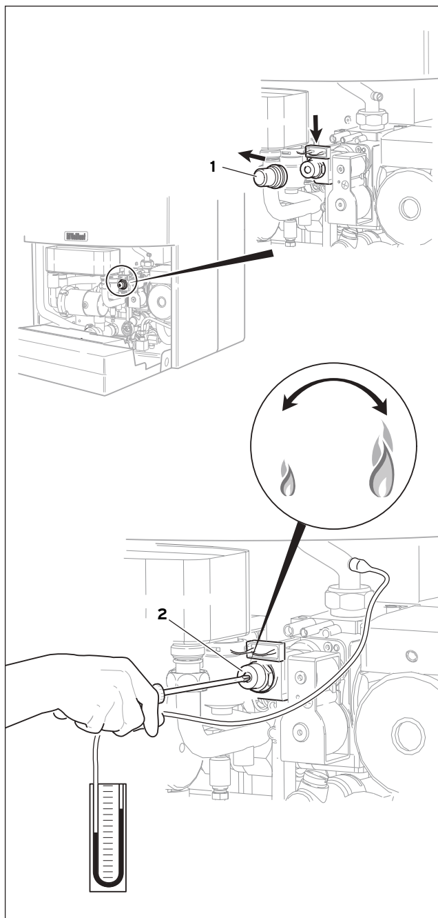
Obr. 5.4: Nastavení startovacího množství plynu Obr. 5.4: Nastavenie zapal'ovacieho množstva plynu 5.4. ábra: A gújtógáz mennyiségének beállítása
