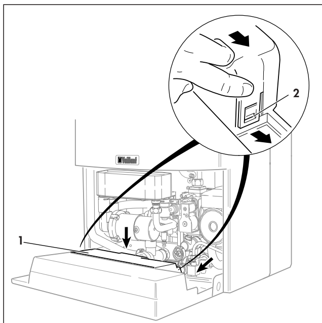
Obr. 3.14: Otevření zadní stěny ovládacího panelu Obr. 3.14: Otvorenie zadnej steny rozvodnej skrinky 3.14. ábra: A kapcsolódoboz hátoldalának kinyitása
