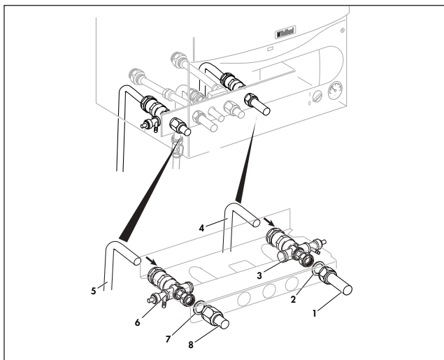
3.11. ábra: A fűtési előremenő és a fűtési visszatérő csatlakozás szerelése HU
