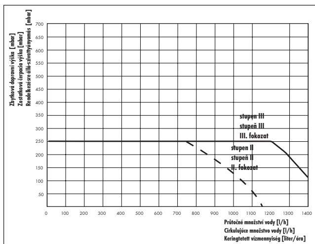
Obr. 7.2: Charakteristika čerpadla
