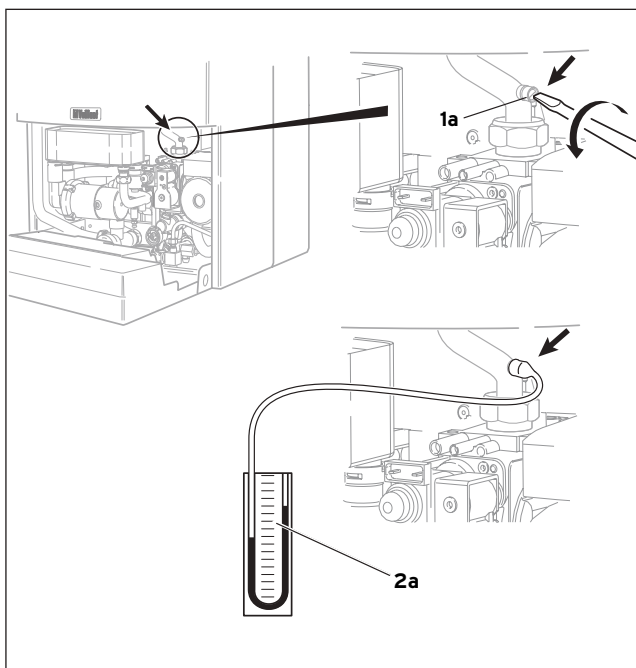
Obr. 5.2: Připojení U-manometru
