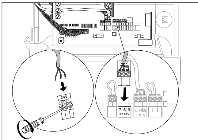
4.7 ábra Hőmérséklet szabályozó csatlakoztatása (7-8-9)
