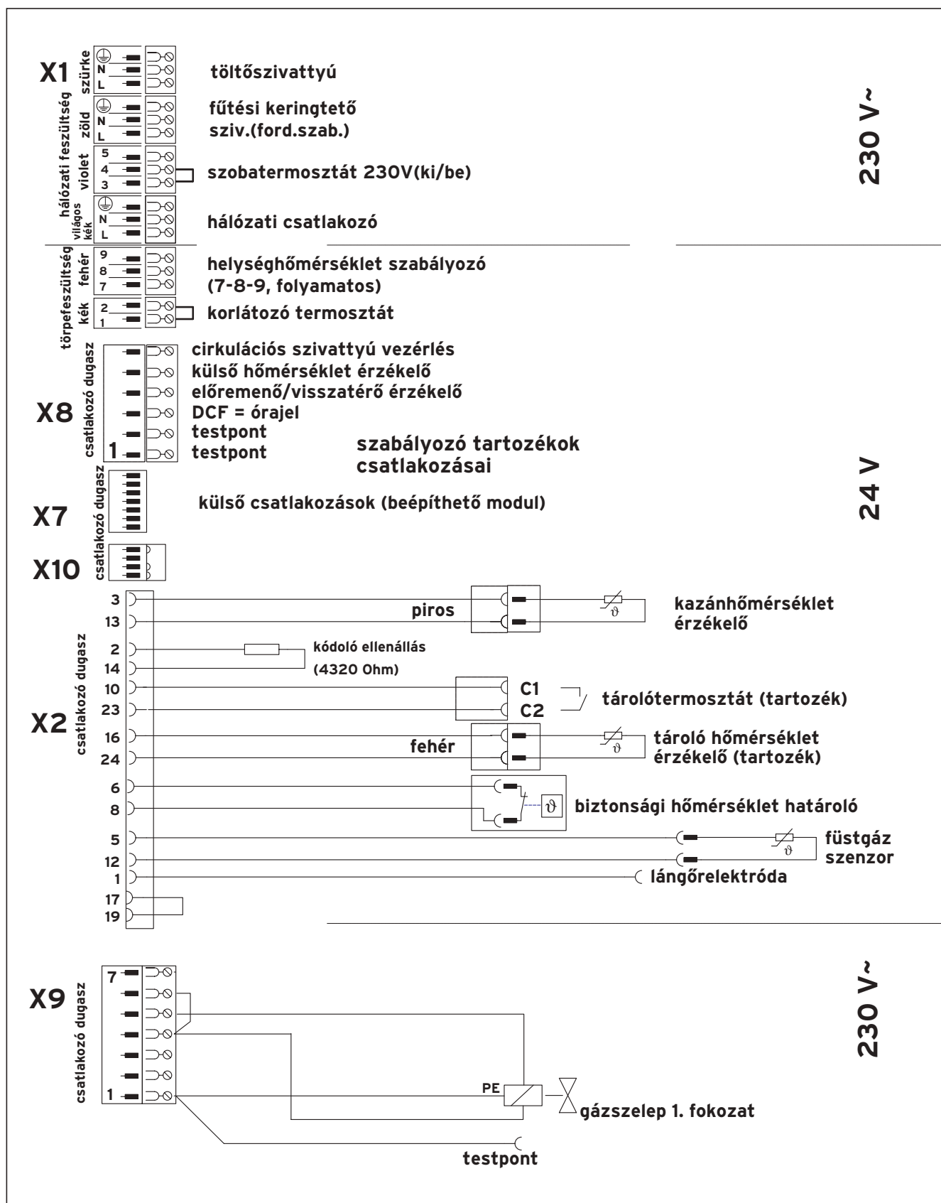
4.5 ábra atmoVIT gázkazán elektromos csatlakozásai.
