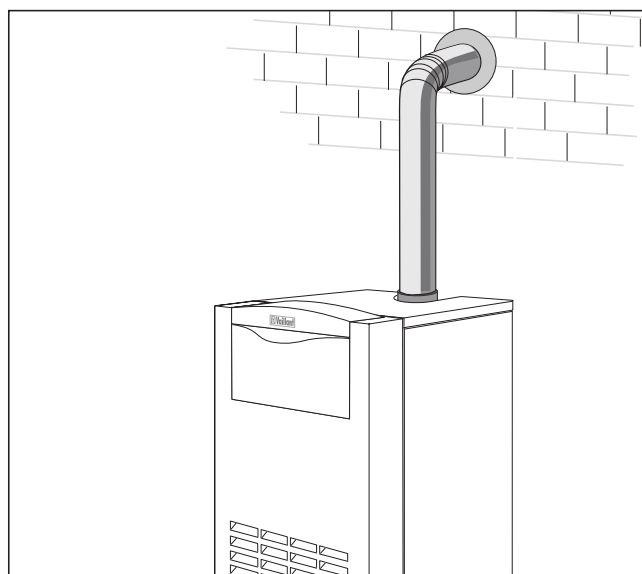
4.3 ábra A füstgázcsonk felszerelése
