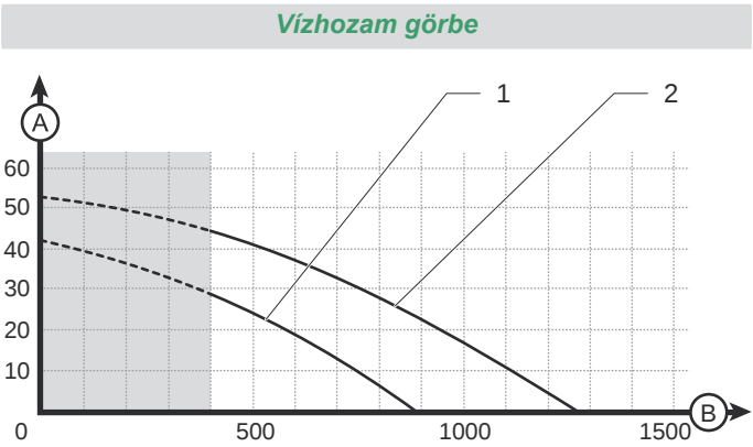
Jelmagyarázat A Nyomás az előremenő és visszatérő fűtőág között (kPa) B Térfogatáram a fűtőkörben (l/h) 1 Fordulatszám min. 2 Fordulatszám max.
