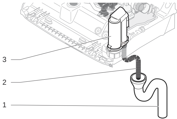
Jelmagyarázat 1 Leeresztő szifon (nem szállított tartozék) 2 Kondenzátum leeresztő tömlő 3 Kondenzátum gyűjtő
