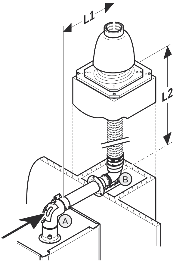
Jelmagyarázat L1 Vízszintes koncentrikus vezeték hossza L2 Függőleges vezeték hossza A Könyök légbevezető nyílással B Bekötő könyök, tartósinnel
