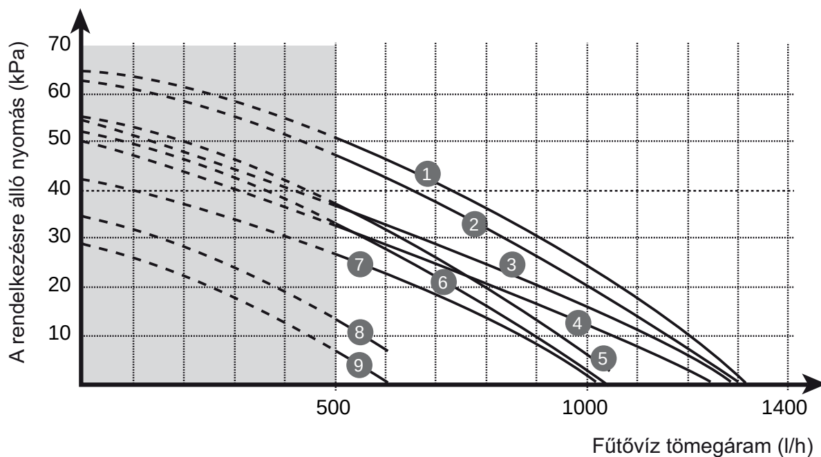
Vízhozam görbe F 30 E
