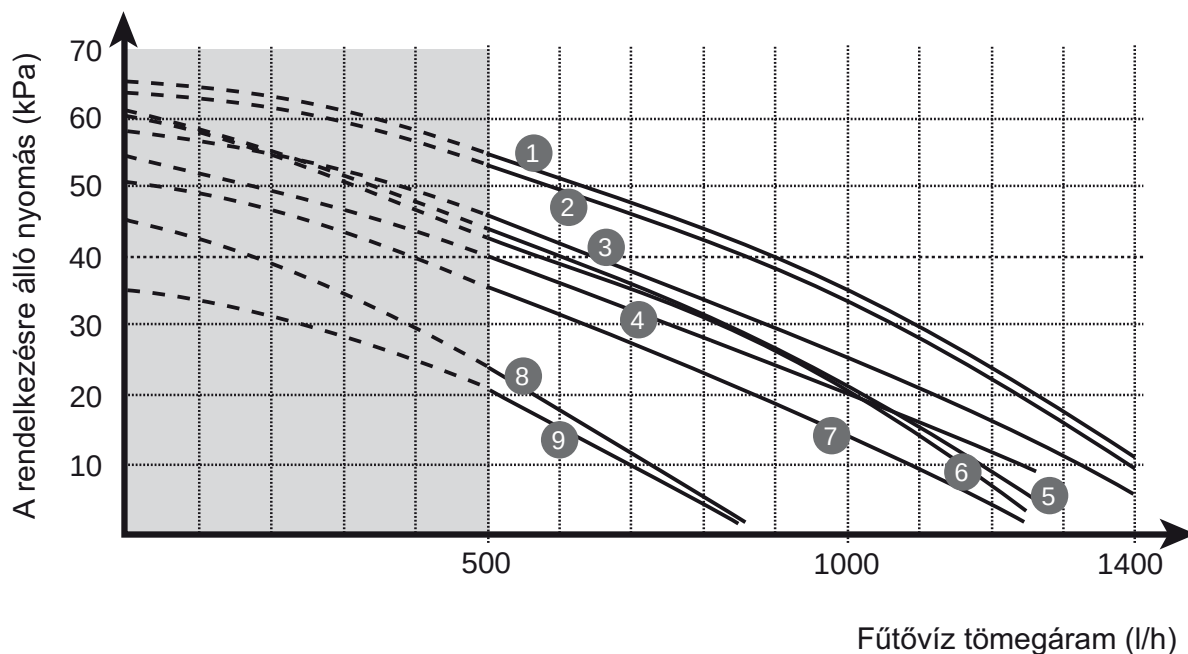
Vízhozam görbe F 35 E
