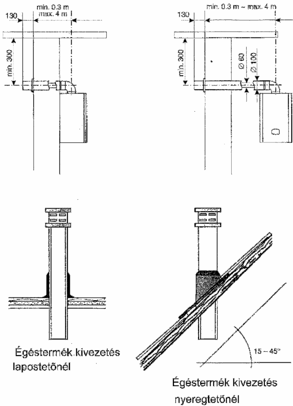
10. ábra Égéstermék kivezetések kialakítása
