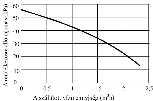
4. ábra Szivattyú jelleggörbe
