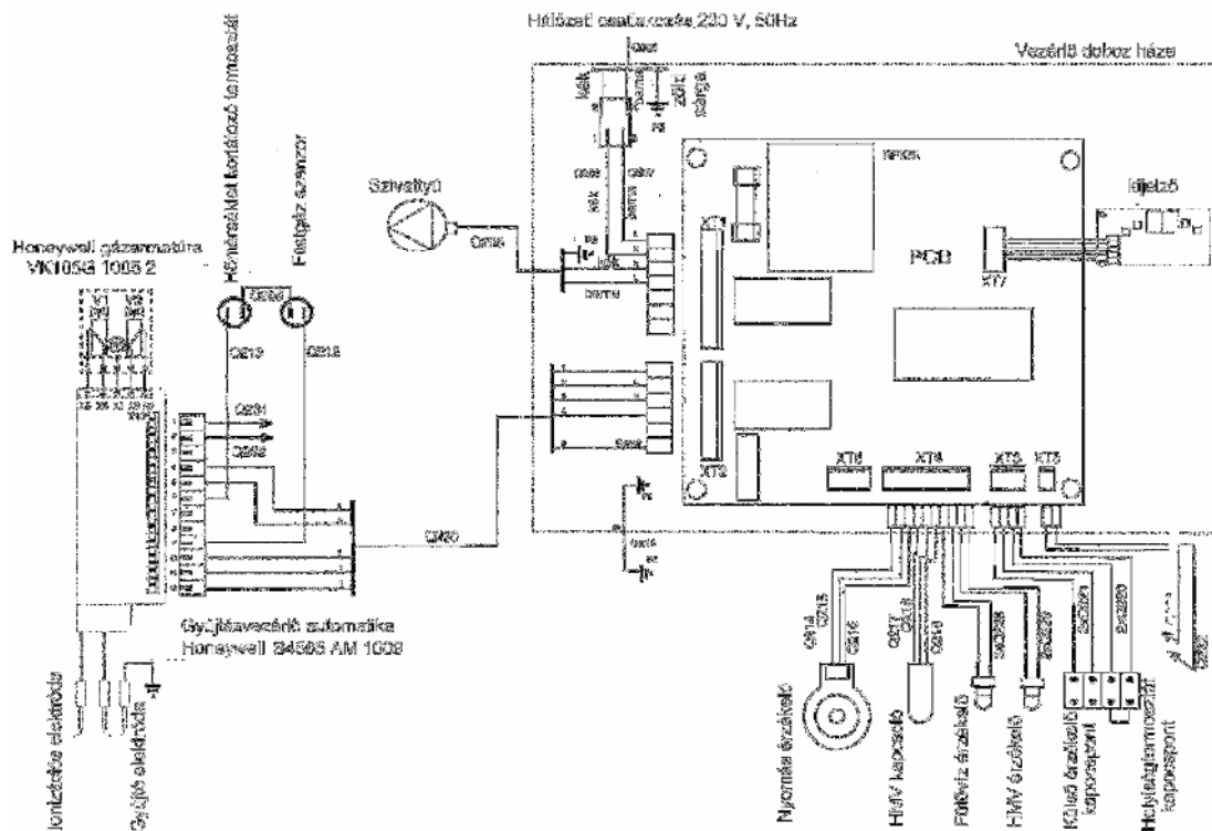
27./b ábra RENOVA C 24 E elektromos kapcsolási rajza
