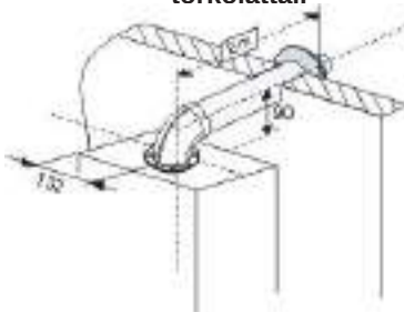
9. ábra C 12 vízszintes égéstermék elvezetés (Ø 60/100)
