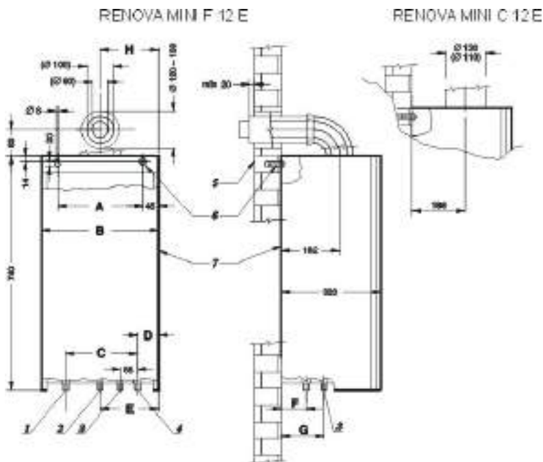
4. ábra A kazán fő- és csatlakozó méretei
