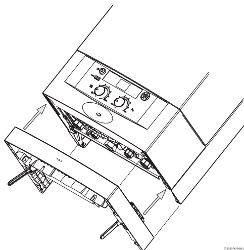
15 ábra A fiók elhelyezése
