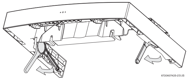
14 ábra Karok felszerelése
