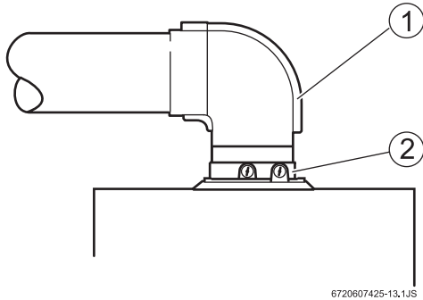
12 ábra Kivezetőkönnyök rögzítése bilinccsel
