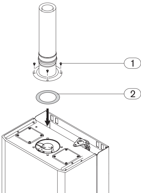
13 ábra Fojtótárca felszerelése
