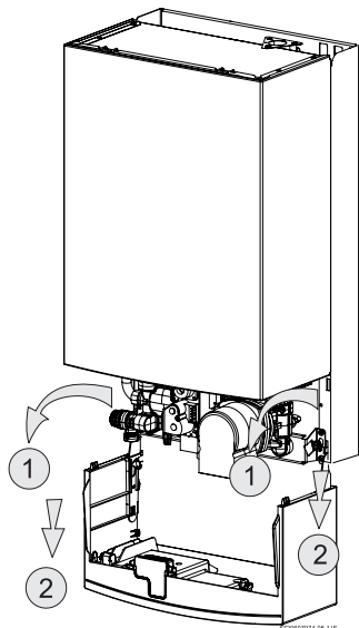
33 ábra Javítási helyzet az elektronikus és vízrészek hozzáféréséhez
