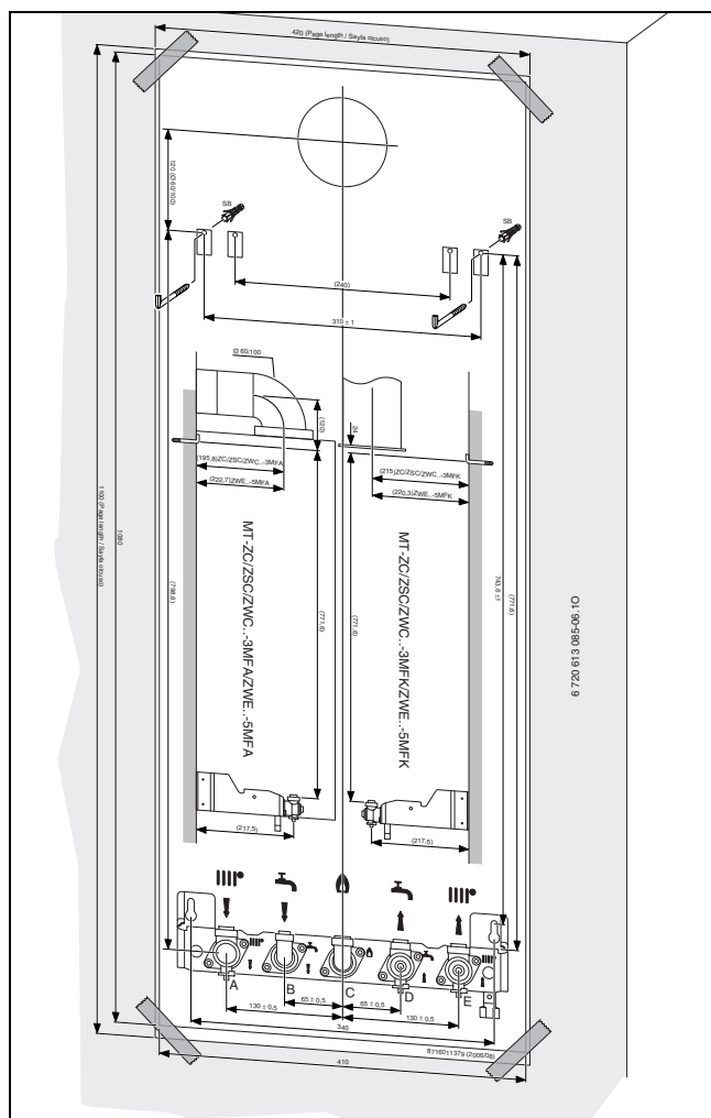
6. ábra Szerelőszablon
