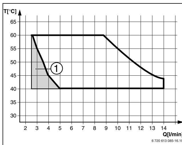
27. ábra +15°C befolyó hidegvíz hőmérséklet diagramm (ZWE 28-5...)
