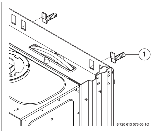
8. ábra A készülék felfüggesztése
