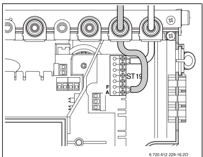
19. ábra Külső érzékelő-csatlakozás
