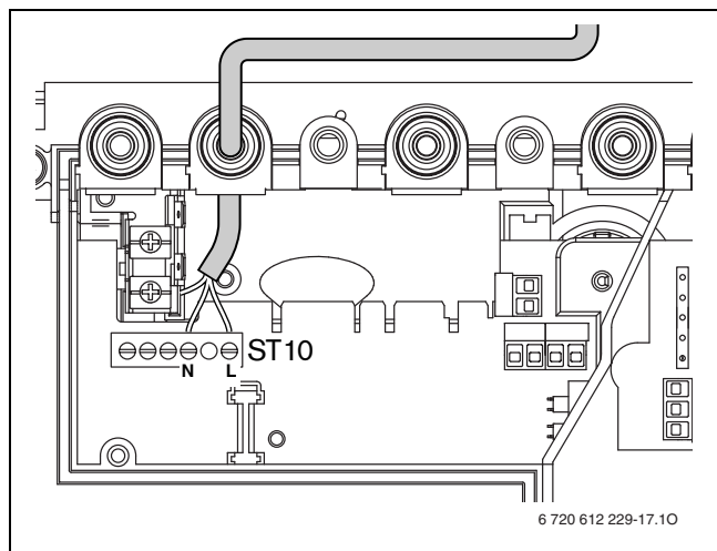
16. ábra ST10-es tápfeszültség ellátó kapocsléc
