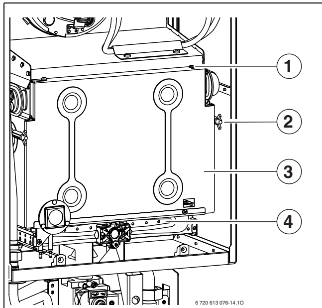
48. ábra Égő nyitása
