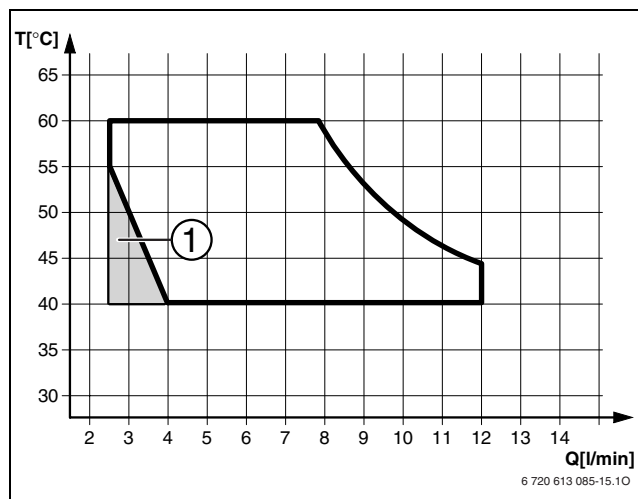
26. ábra +15°C befolyó hidegvíz hőmérséklet diagramm (ZWE 24-5...)
