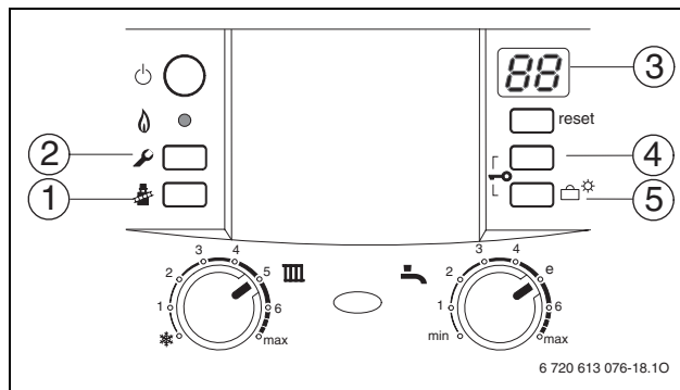
35. ábra A kezelő elemek áttekintése
