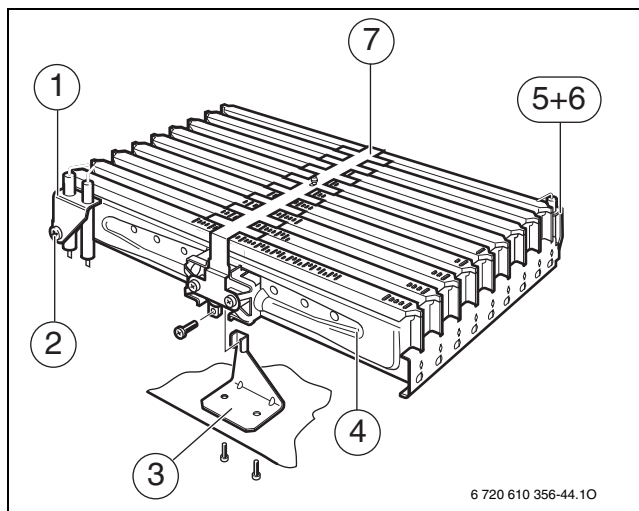
49. ábra Égő részegység
