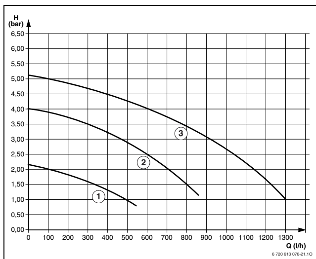
33. ábra ZWE 28-5 (szerelő csatlakozáslap nélkül) szivattyú jelleggörbék
