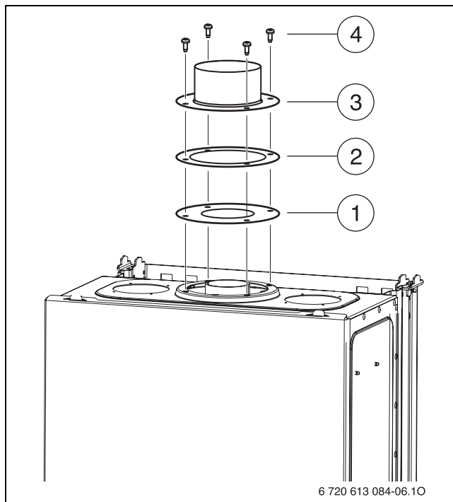
11. ábra Füstgáztartozék rögzítése
