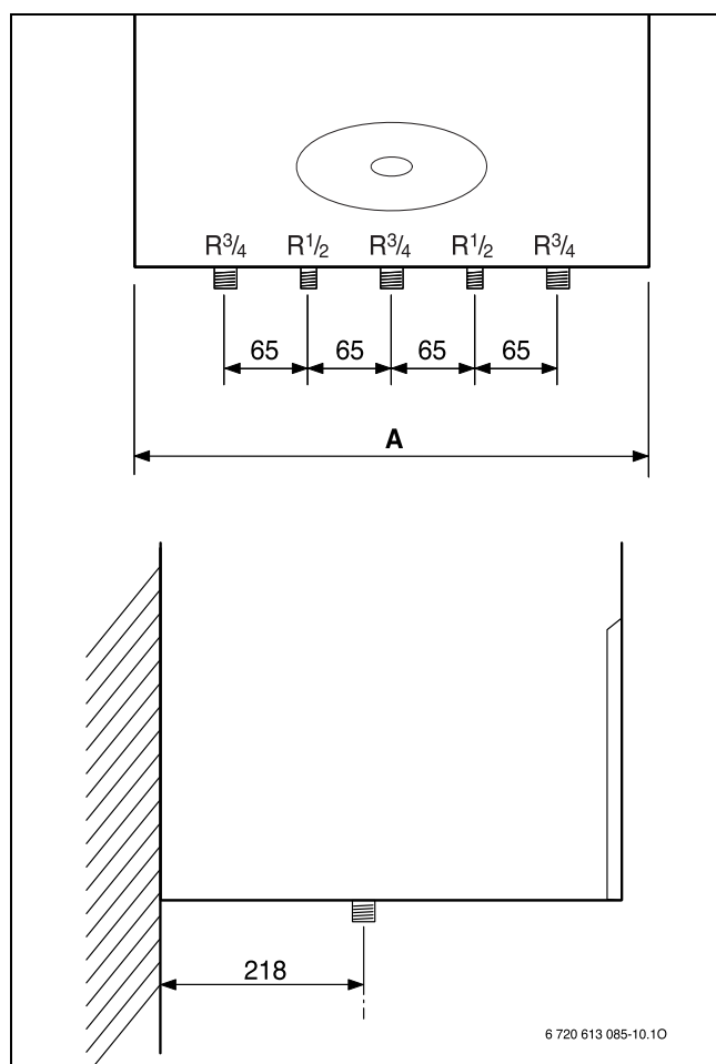
12. ábra Csatlakozási méretek
