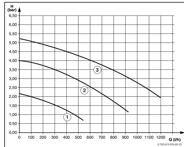
32. ábra ZWE 24-5 (szerelő csatlakozáslap nélkül) szivattyú jelleggörbék
