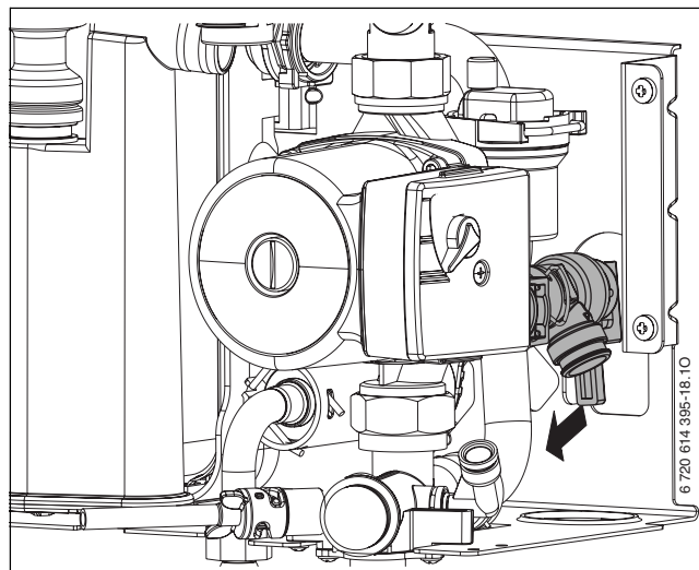
66 ábra Biztonsági szelep (fűtési kör)
