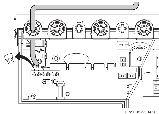
20 ábra Easyswitch csatlakozás
