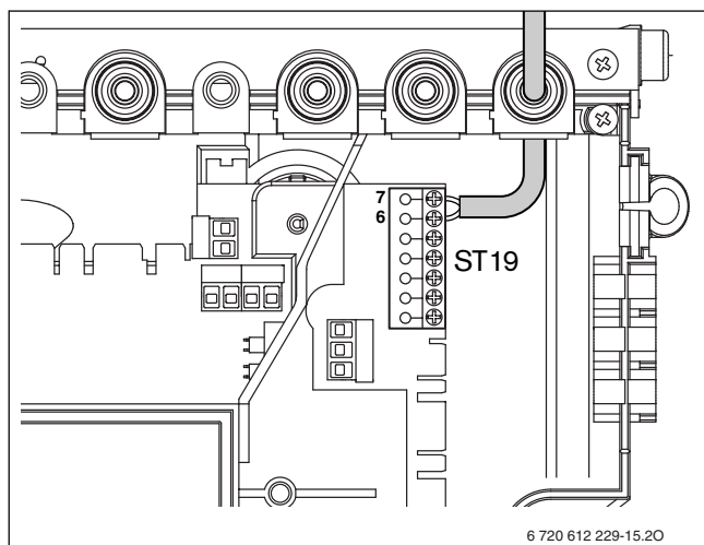
21 ábra Szabályozó csatlakozás
