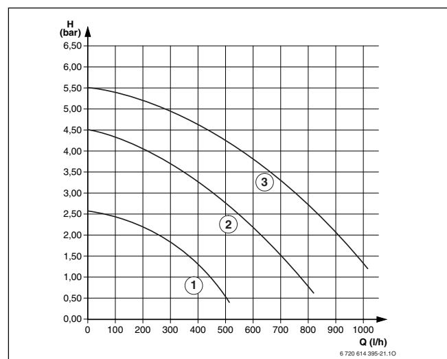
43 ábra Szivattyú-jelleggörbék (szerelőpanel nélkül)
