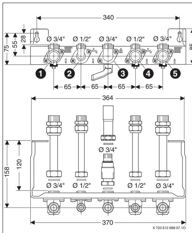
7 ábra Szerelőpanel (külön rendelhető tartozék)
