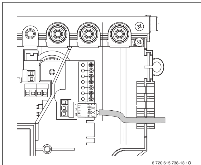
24 ábra A melegvíztároló hőmérséklet érzékelőjének (NTC) csatlakozása
