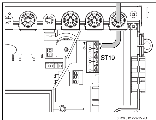
23 ábra Az EMS-buszmódul csatlakozása
