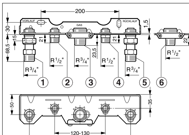
8 ábra Összekötő lemez a vízszintes szereléshez
