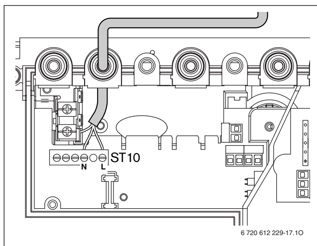
30 ábra ST10-es tápfeszültség ellátó kapocsléc
