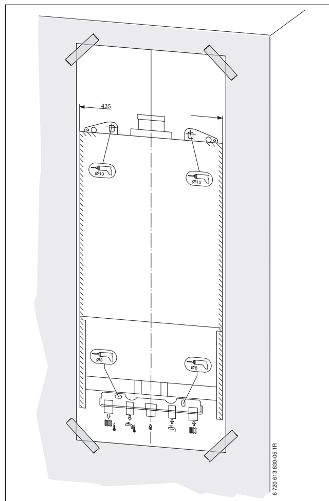
6 ábra Szerelősablon
