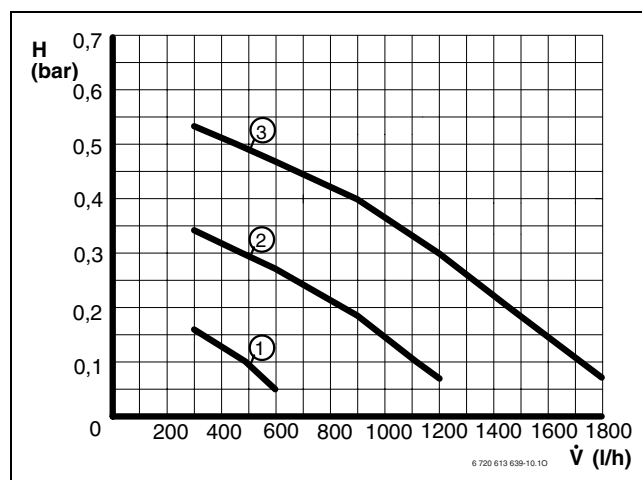
26. ábra Szivattyú-jelleggörbék
