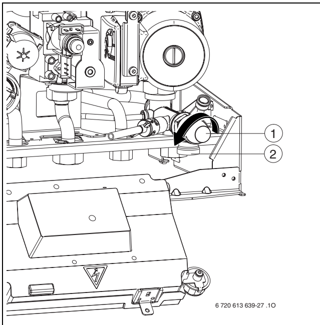
39. ábra Biztonsági szelep
