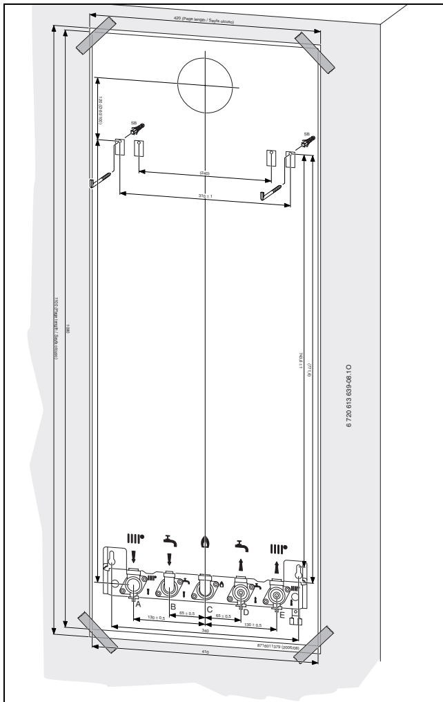
7. ábra Szerelő sablon (példa)
