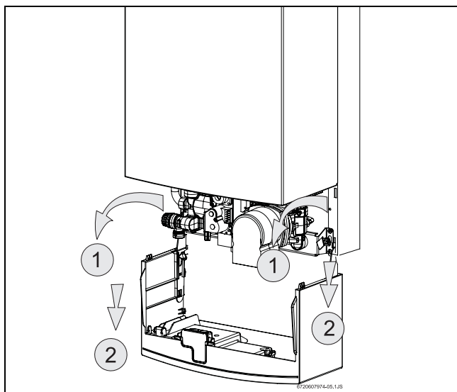
30. ábra Javítási helyzet az elektronikus és vírzészek hozzáférésehez
