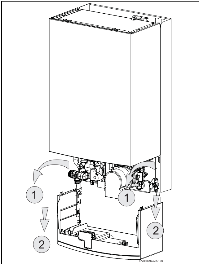
9. ábra Javítási helyzet a víz- és elektromos rendszer hozzáférése céljából
