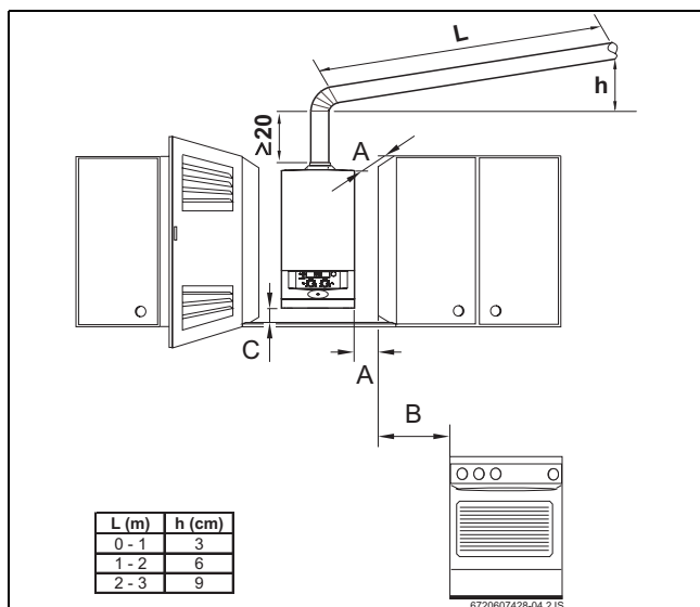
6. ábra Minimális oldaltávolságok
