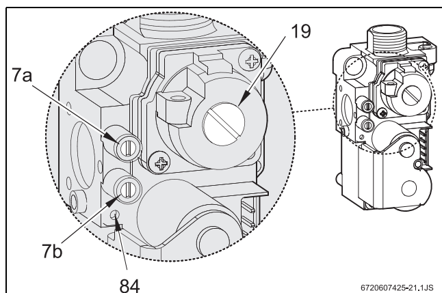
27. ábra Gázszelep
