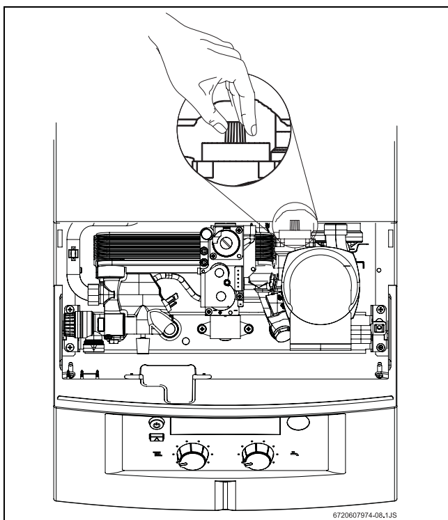
14. ábra Légtelenítő
