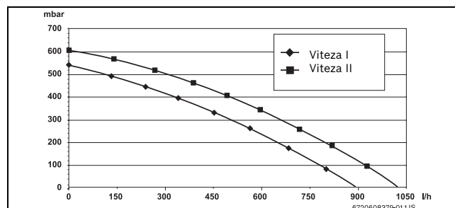
5. ábra A szivattyú jelleggörbéje
