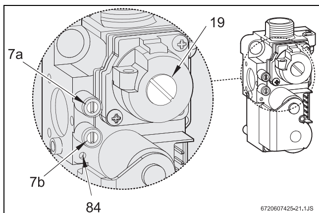
30 ábra Gázszelep
