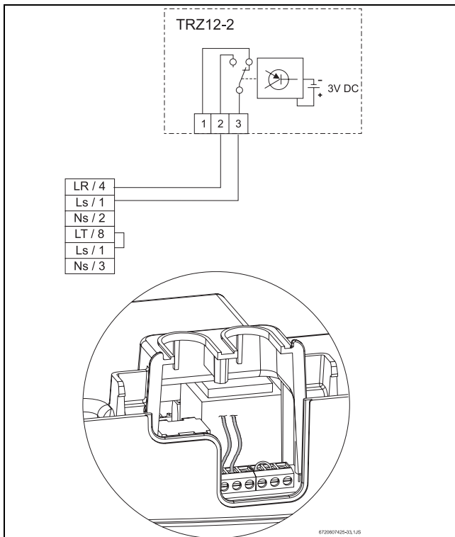
20 ábra TRZ 12 - 2
