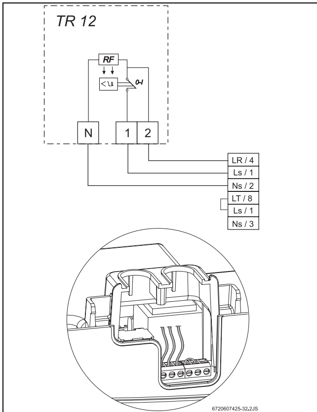
19 ábra TR 12
